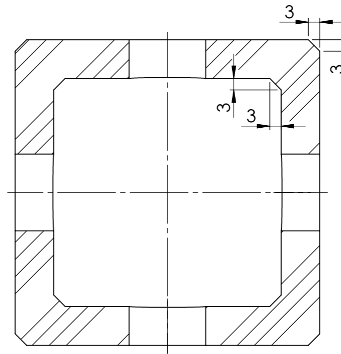
SCHNITT C-C
